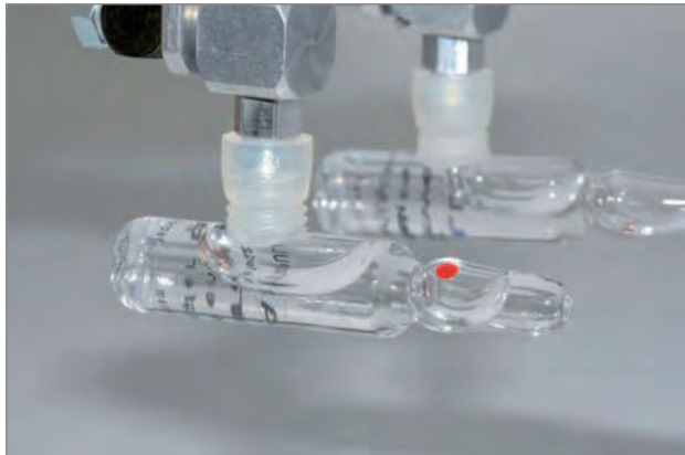
硅橡胶制成的波纹吸盘TGB应用于搬运医用安瓿
